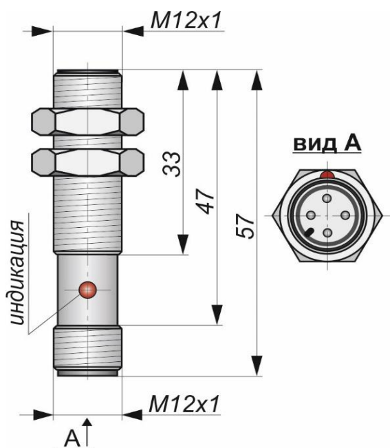
Габаритный чертеж
